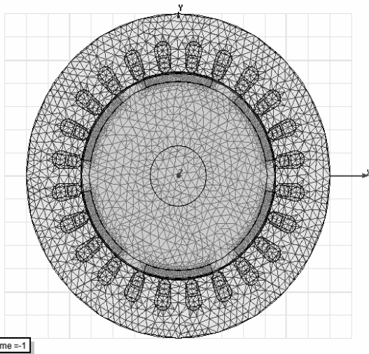
شکل ۴ مش مدل دوبعدی موتور
