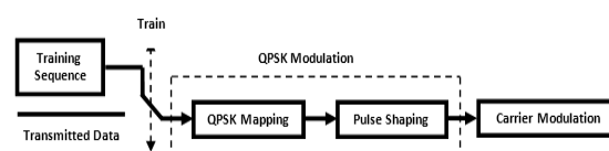
شکل ۱۰ بلوک دیگرام فرستنده
