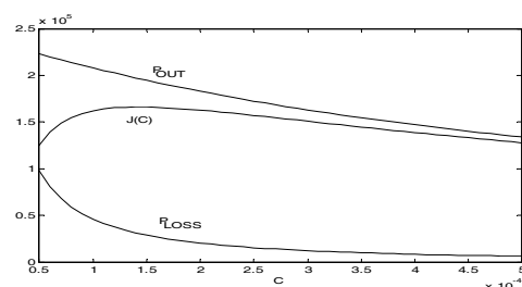
شکل ۳ نمودارهای توان خروجی ( P_{out} )، توان تلفاتی ( P_{loss} )
