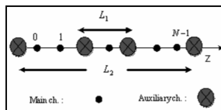
شکل ۹ آرایه خطی با چهار کانال کمکی
