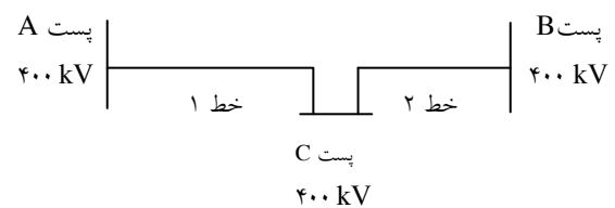
شکل ۲ خط تک‌مداره‌ای که در پست میان‌راهی وارد - خارج شده است
