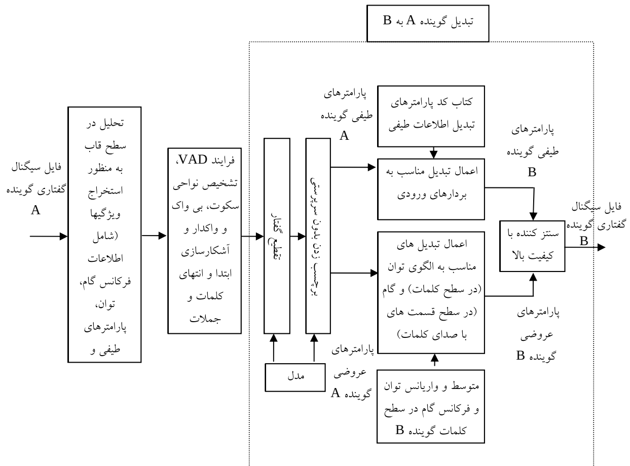
شکل ۶: بلوک دیاگرام سیستم جدید تبدیل گفتار
