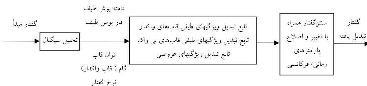
شکل ۵ بلوک دیاگرام مورد استفاده در سیستم تبدیل گفتار برای روش GMM_VC
