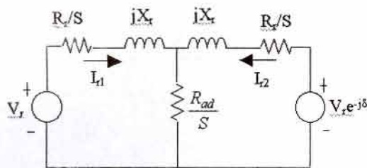
شکل ۴ مدار معادل سلسین دو موتور
