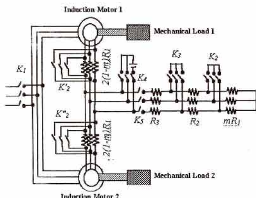
شکل ۵ ساختار سلسین دو موتور اصلاح شده
