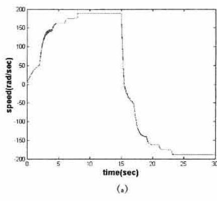
شکل ۷ نتایج شبیه‌سازی برای راه‌اندازی و معکوس کردن سرعت، الف- سرعت دو موتور مستقل، ب- زاویه بین رتور دو موتور مستقل، ج- سرعت دو موتور در سلسین سستی، د- زاویه بین دو رتور در سلسین سستی، ه- سرعت دو موتور در سلسین اصلاح شده، و- زاویه بین دو رتور در سلسین اصلاح شده.
