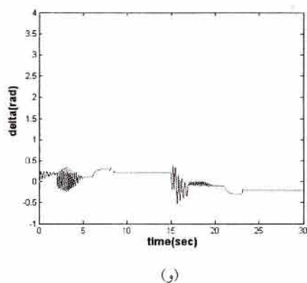
شکل ۷ نتایج شبیه‌سازی برای راه‌اندازی و معکوس کردن سرعت، الف- سرعت دو موتور مستقل، ب- زاویه بین رتور دو موتور مستقل، ج- سرعت دو موتور در سلسین سستی، د- زاویه بین دو رتور در سلسین سستی، ه- سرعت دو موتور در سلسین اصلاح شده، و- زاویه بین دو رتور در سلسین اصلاح شده.
