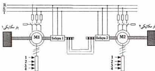
شکل ۱ طرح اتصال سلسین چهار موتور
