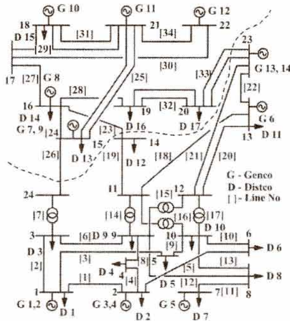
شکل ۷ شبکه ۲۴ باسه IEEE-RTS
