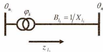
شکل ۲ جابه‌جاگر فاز ایده‌آل، بر روی شاخه l_1
