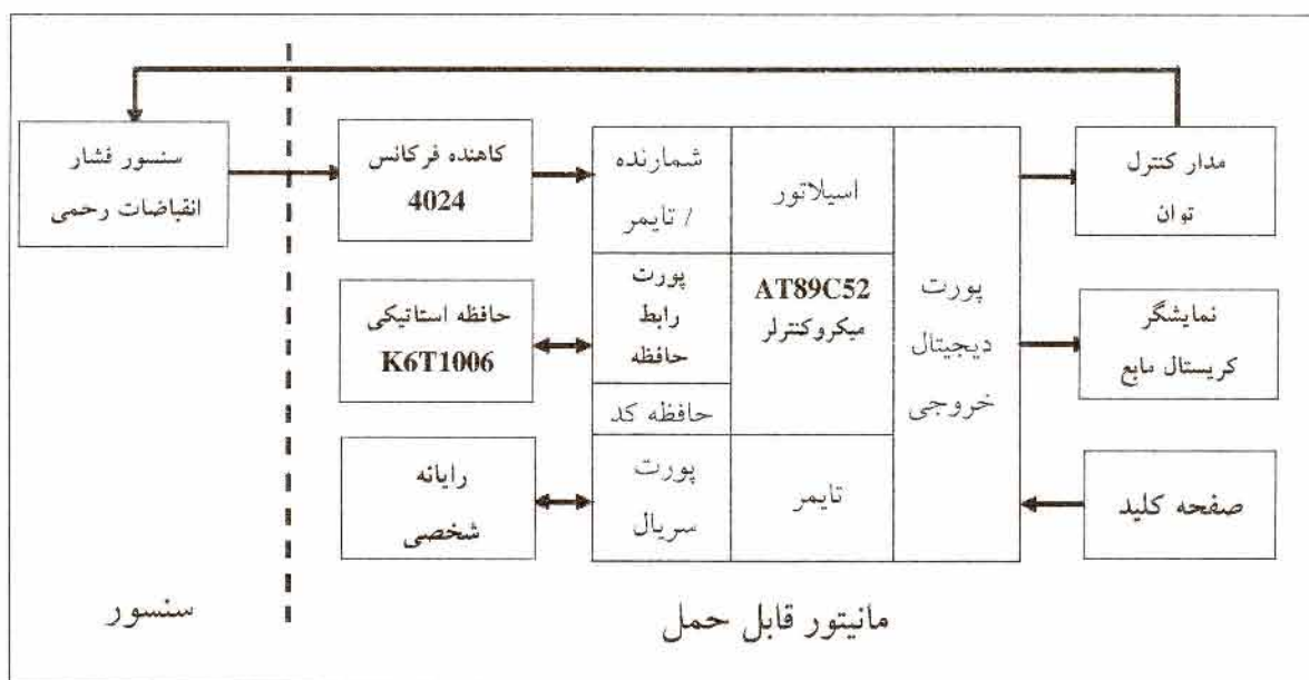
شکل ۱ بلوک دیاگرام سیستم پیشنهادی
