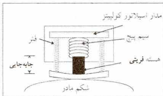
شکل ۲ ساختمان سنسور
