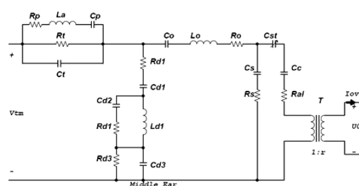
شکل ۴ مدل الکتروآکوستیکی گوش میانی [۷]
