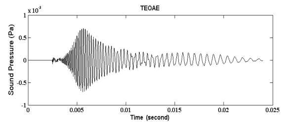
شکل ۸ سیگنال CEOAE شبیه سازی شده با مدل جدید
