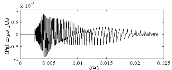
شکل ۹ سیگنال CEOAE شبیه سازی شده با مدل اولیه [۷]
